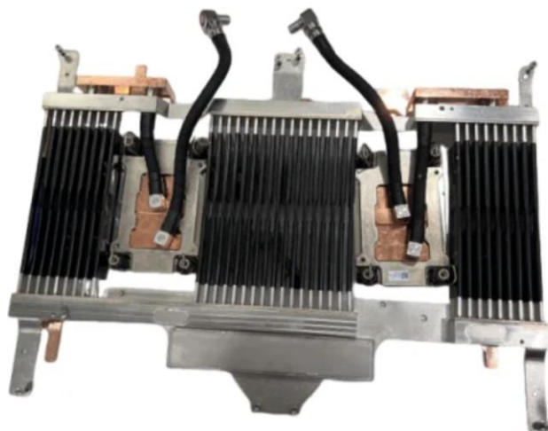
圖表一、Dimm Coldplate
